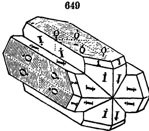
Andreasberg.
